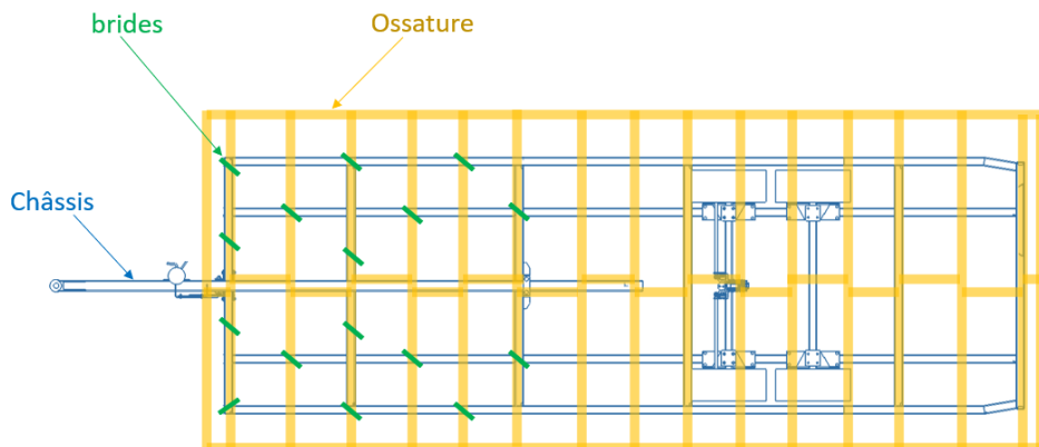
Vue exemples de positionnements de brides
